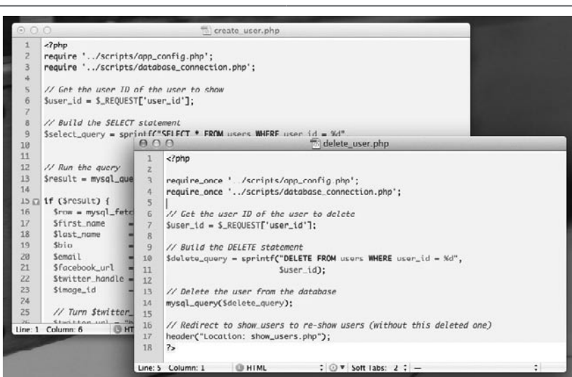
Рис. 10.5. При достаточно большом экране лучше всего при вырезке, копировании и вставке просматривать сразу два кодовых фрагмента, расположив их рядом
