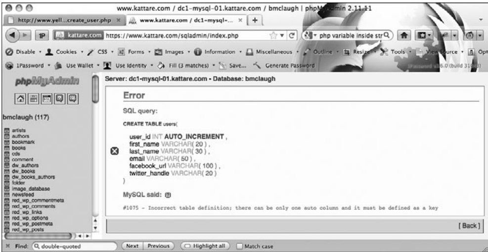
Рис. 6.2. Ошибка в phpMyAdmin
