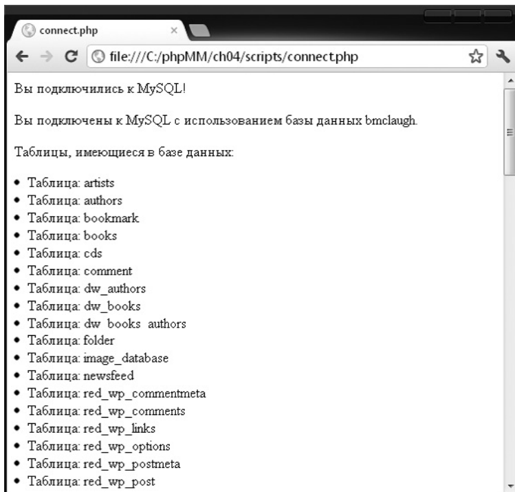
Рис. 4.5. Результат работы сценария connect.php
