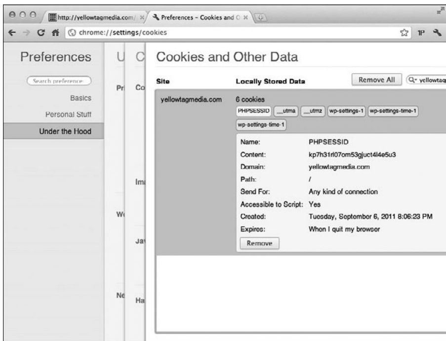
Рис. 13.7. Без cookie-файлов не обойтись, но вам все же удастся при этом избежать хранения на машине клиента какой-либо ценной информации
