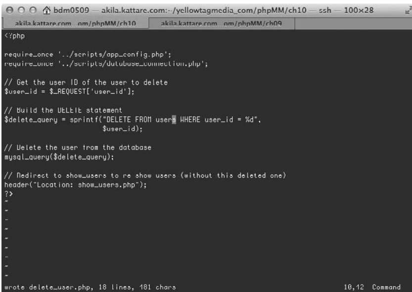
Рис. 10.6. При ограниченном пространстве экрана или если вы предпочитаете работать с более компактными формами, воспользуйтесь вкладками своего редактора (здесь показан Terminal компьютера Mac)
