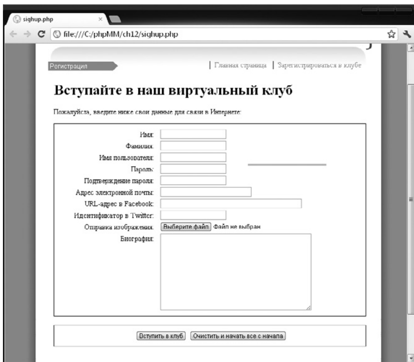
Рис. 12.11. Меню на странице первоначальной регистрации
